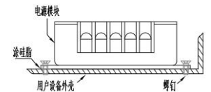
马蹄孔封装安装方式
