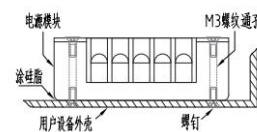
常规安装方式
